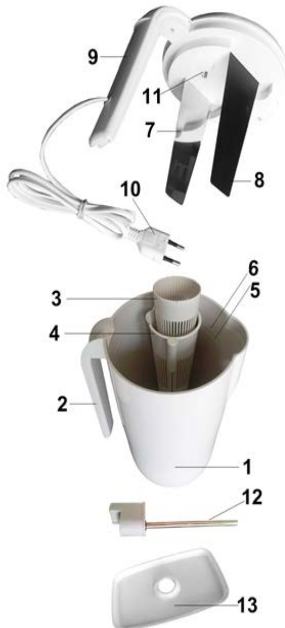
1.zīm. Konstrukcija
